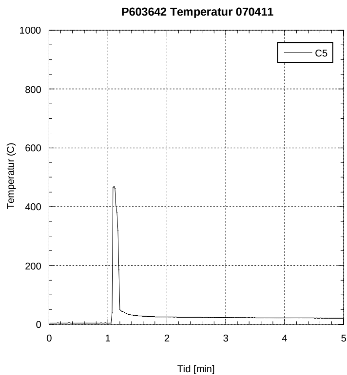
Diagram 7 Vägtemperaturer i cisternen efter antändning
