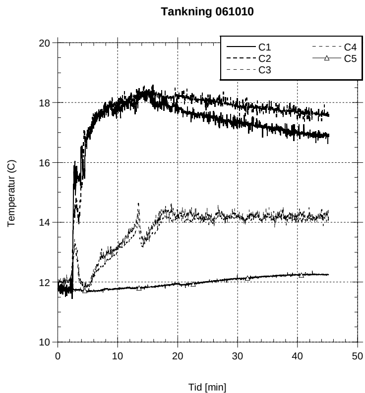
Diagram 1 Uppmätt temperatur vid fyllningen av cisternen
