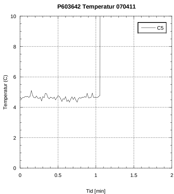
Diagram 5 Vägtemperaturer i cisternen fram till antändning
