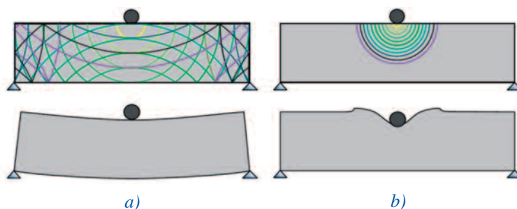
Figur 3: Vågutbredning och strukturens respons för a) långsam respektive b) mycket snabb belastning.
