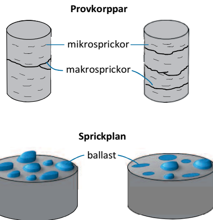
Figur 5: Schematisk bild av den dynamiska inverkan på sprickbildningen i enaxiellt drag. Till vänster: långsam belastning, till höger: snabb belastning.
