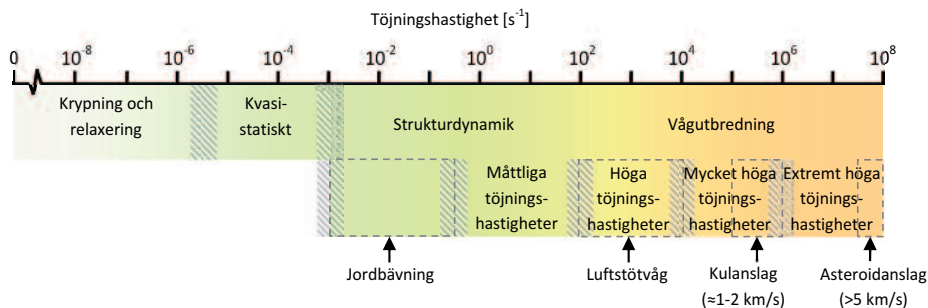
Figur 2: Töjningshastighetens inverkan på problembeskrivningen; efter bland annat Zukas (2004) och Ramesh (2008).
