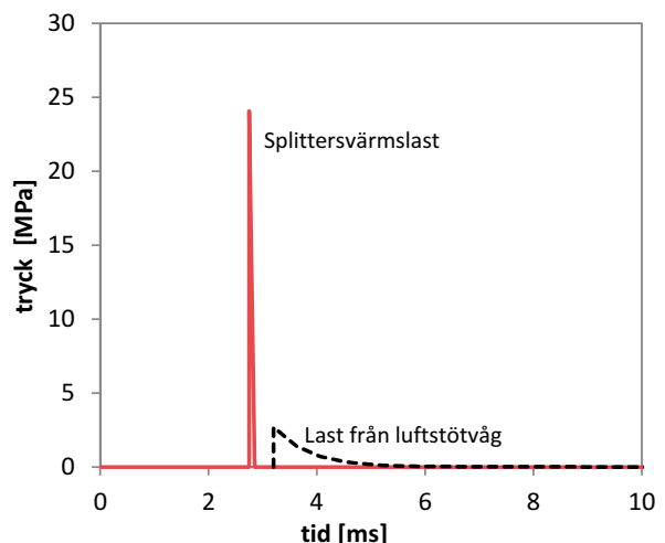
Figur 1: Idealiserad explosionsbelastning från arkivbomben.
