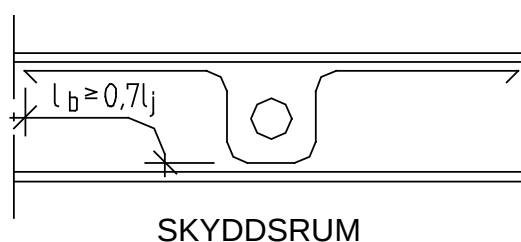
Figur 3:44a. Armeringsutformning med förankringslängd l_b vid ingjutning av rör i stomkonstruktionen
