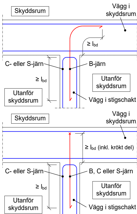
Figur 6:42f. Schematisk illustration av armeringsutformning vid anslutning av vägg i stigschakt till skyddsrummets begränsningsvägg.
