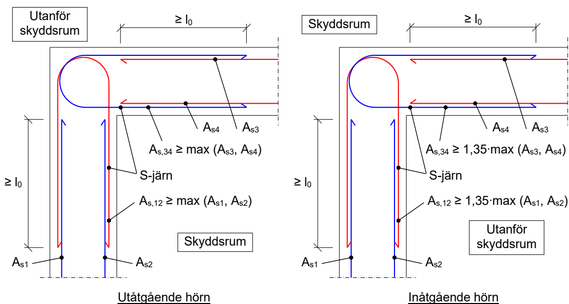
Figur 6:42b. Schematisk illustration av armeringsutformning vid anslutning inom hörnområde.
