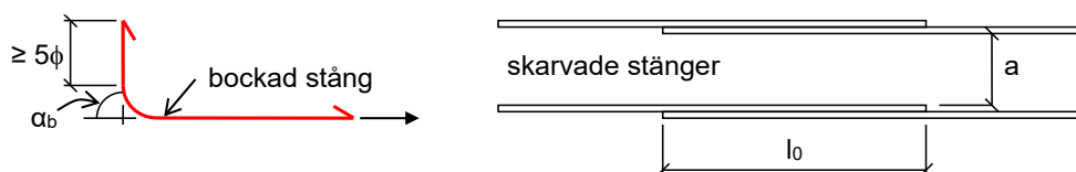
Figur 6:41a. Definition av bockningsvinkel \alpha_b och fritt avstånd a mellan stänger.
