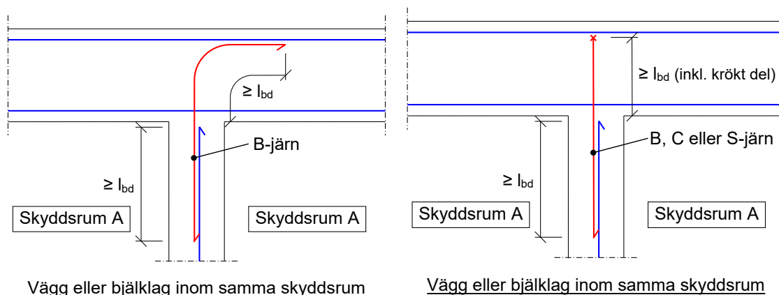
Figur 6:42e. Schematisk illustration av armeringsutformning vid anslutning till rak konstruktionsdel med enkellarmerat utförande inom samma skyddsrum.
